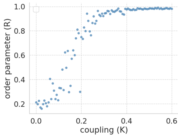
Рис. 1. Изменение параметра порядка при N=25 от параметра K в связях с симплексами первого порядка.
